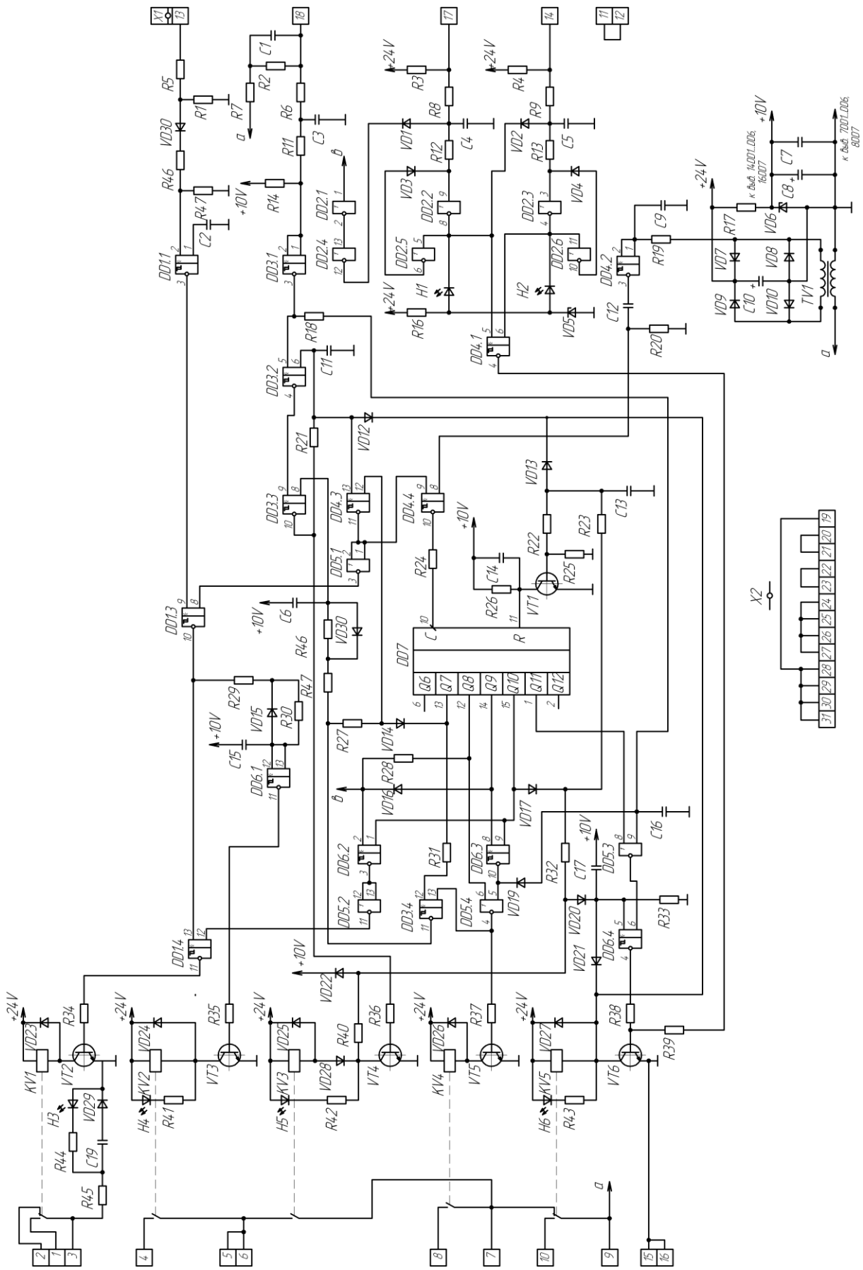
Рисунок 16 – Схема электрическая принципиальная блока управления горелкой ГБ
