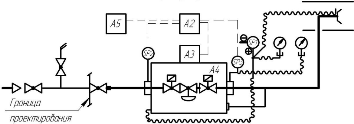
Рисунок 3 – Схемы функциональные
